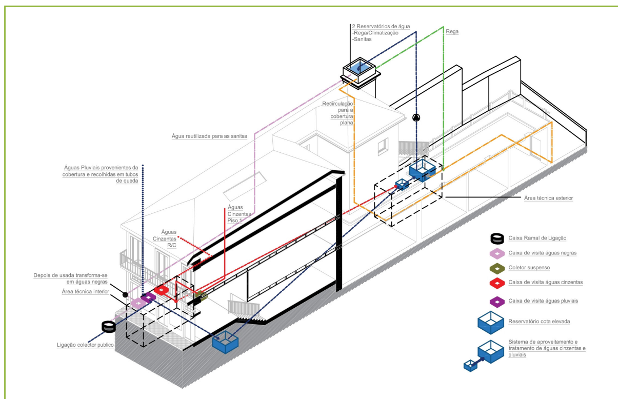
Fig. 11. Esquema representativo da gestão das águas.
