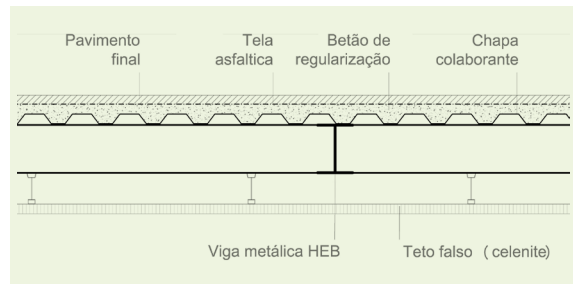
Fig. 31. Pormenor laje colaborante.
