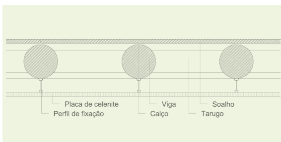
Fig. 30. Pormenor da Laje de piso a aplicar.
