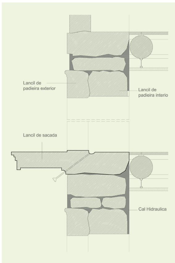
Fig. 18. Pormenor parede de tabique simples.
