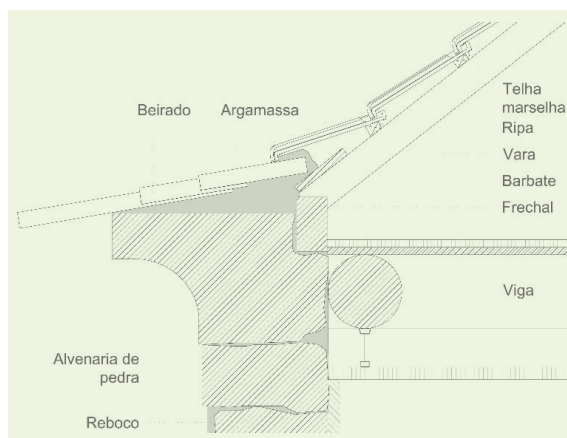
Fig. 41. Pormenor de beirado.
