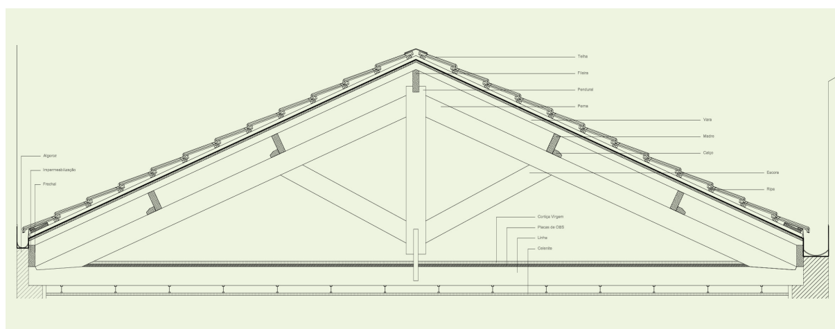
Fig. 32. Exemplo de cobertura típica da época e existente no caso de estudo.
