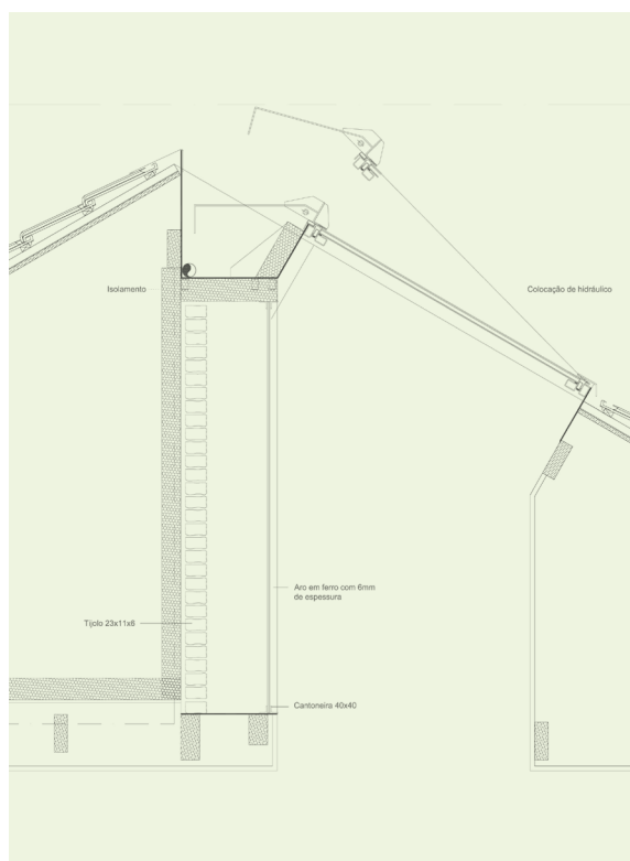
Fig. 35. Pormenor claraboia com parede de trombe.
