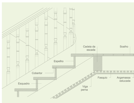
Fig. 36. Pormenor construção de uma escada.
