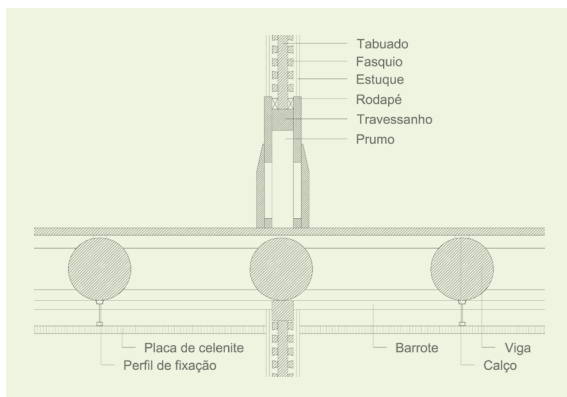
Fig. 19. Pormenor de parede exterior.
