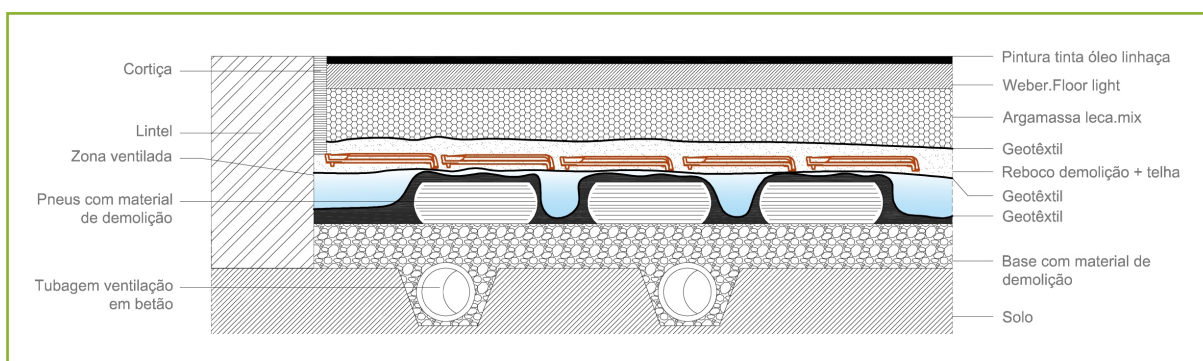
Fig. 20. Solução adotada para laje de pavimento da cave.
