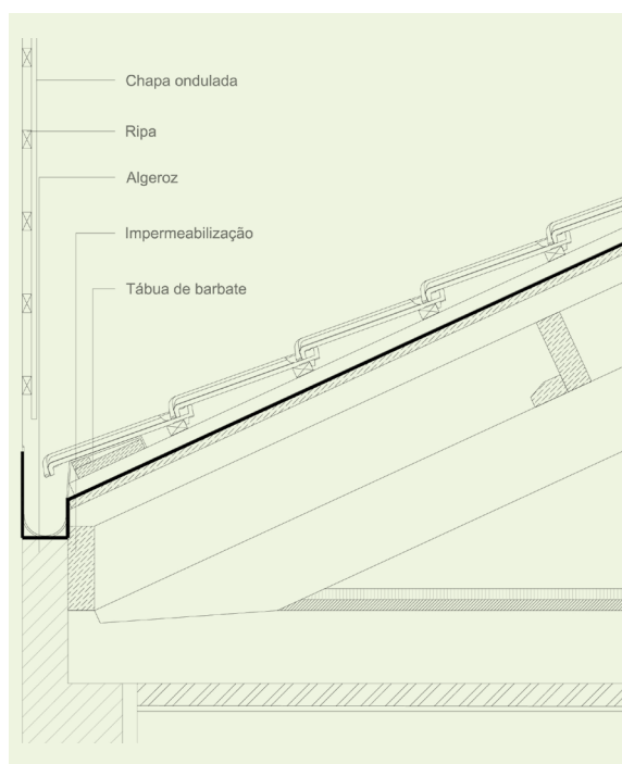
Fig. 40. Pormenor do algeroz.
