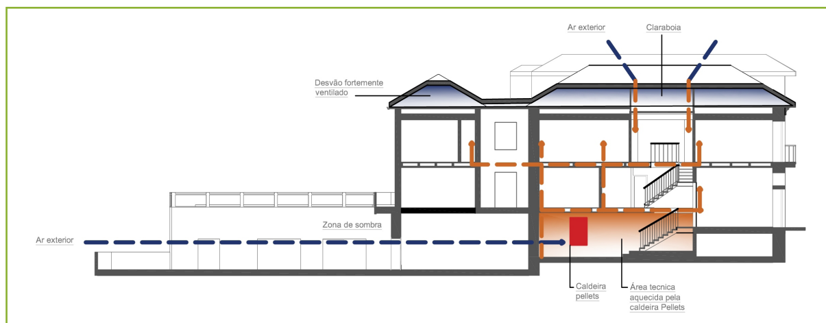
Fig. 10. Funcionamento das ventilações no corpo principal do edifício.
