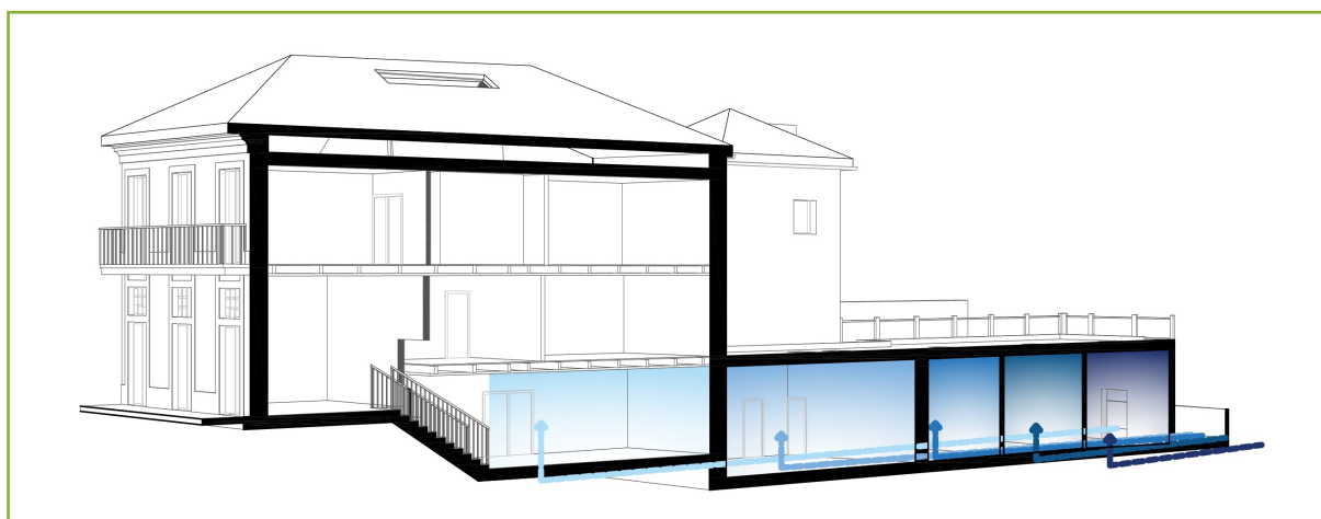
Fig. 9. Funcionamento das ventilações no corpo 3 e compartimentos no seu alinhamento.
