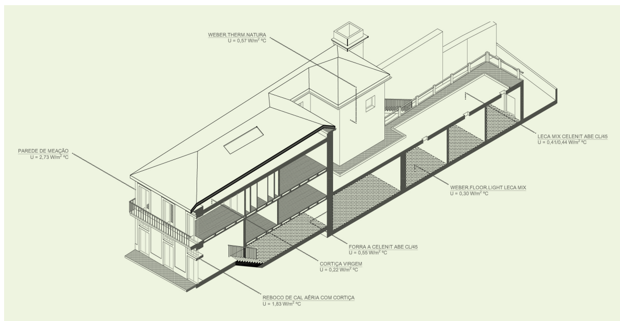
Fig. 8. Perspetiva com o valor do coeficiente de condutibilidade térmica dos elementos principais.
