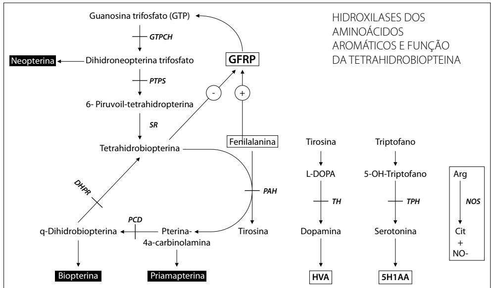
Figura 2. Esquema representativo da síntese de BH4. (Adaptada de Blau, N [2005]).
