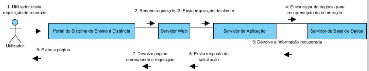
Figura 17 – Diagrama de Colaboração do Sistema
