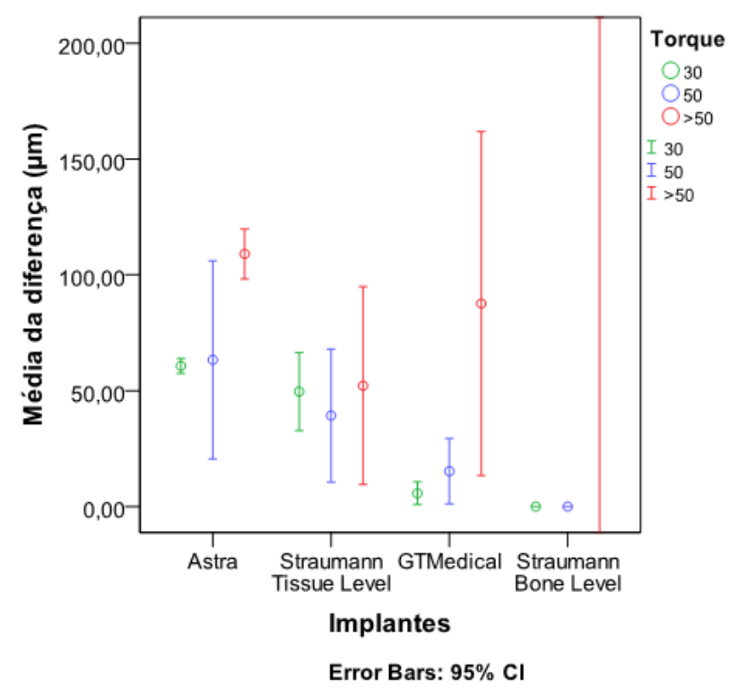
Figura 26 - média da deformação ( \mu\text{m} ) produzida pela aplicação dos implantes das marcas Astratech TM , GTMedical e Straumann Tissue level ® , com 3 torques de inserção (o círculo indica a média de deformação e a barra o respetivo intervalo de confiança).
