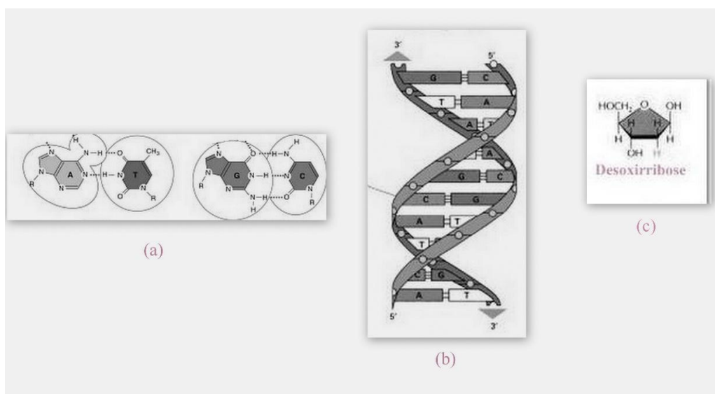
Figura 3: Estrutura do DNA: (a) ligação entre as bases; (b) dupla cadeia; (c) pentose (Adaptado de (Tropp, 2012; Alberts et al. , 2006)).
