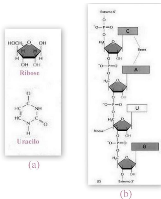
Figura 2: Estrutura do RNA: (a) Ribose e Uracilo; (b) cadeia linear. (Adaptado de (Alberts et al. , 2006)).
