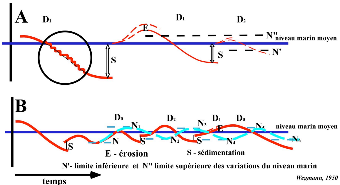
Fig. 1- Représentation graphique de la composante verticale des mouvements orogéniques. En A, la sédimentation et la subsidence sont plus au moins en équilibre. En B, la sédimentation n'est pas assez forte pour compenser la subsidence. Dans le cercle, il est montré l'agrandissement de la courbe qui, bien que continue en apparence, est en fait composée d'une suite de mouvements saccadés (voir texte).
