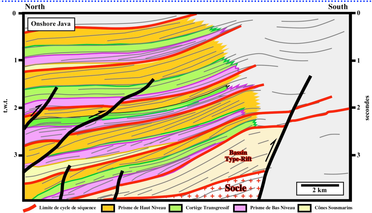
Fig. 3- Dans cette interprétation, les registres stratigraphiques soulignent des épisodes tectoniques saccadés qui étant à la limite de la résolution de la biostratigraphie peuvent amener les explorateurs non avertis à considérer le raccourcissement des sédiments comme polyphasé à la suite des différents régimes tectoniques. Une telle interprétation aurait inévitablement des conséquences dans la datation des pièges potentiels.
