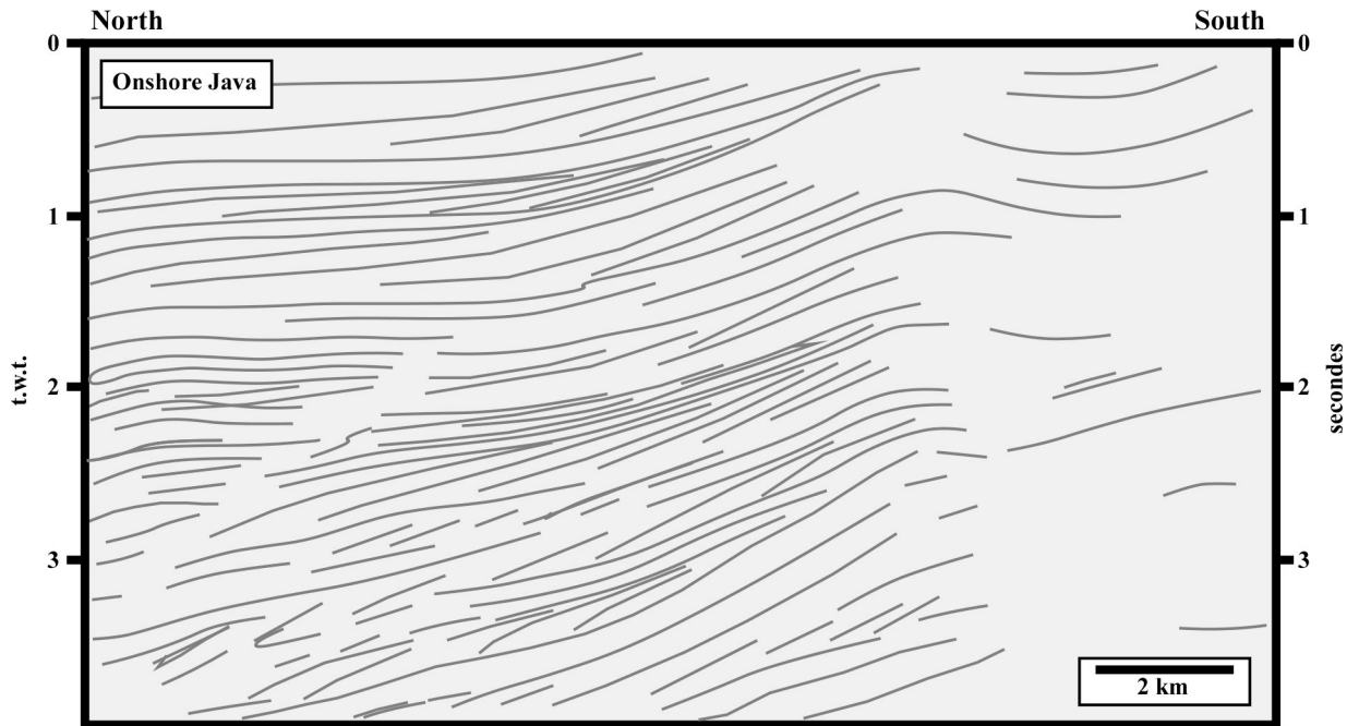
Fig. 2- Sur cette ligne, un géologue doit-il considérer le raccourcissement des sédiments comme épisodique et récent, autrement dit, postérieur à la migration des hydrocarbures, ou doit-il considérer que le raccourcissement est en continu et qu'il a démarré dès le début du bassin de type-rift?
