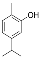
Figura 6 - Fórmula química estrutural do carvacrol, um constituinte do óleo de orégão, e que tem propriedades anti-séticas (Pubchem, 2014).
