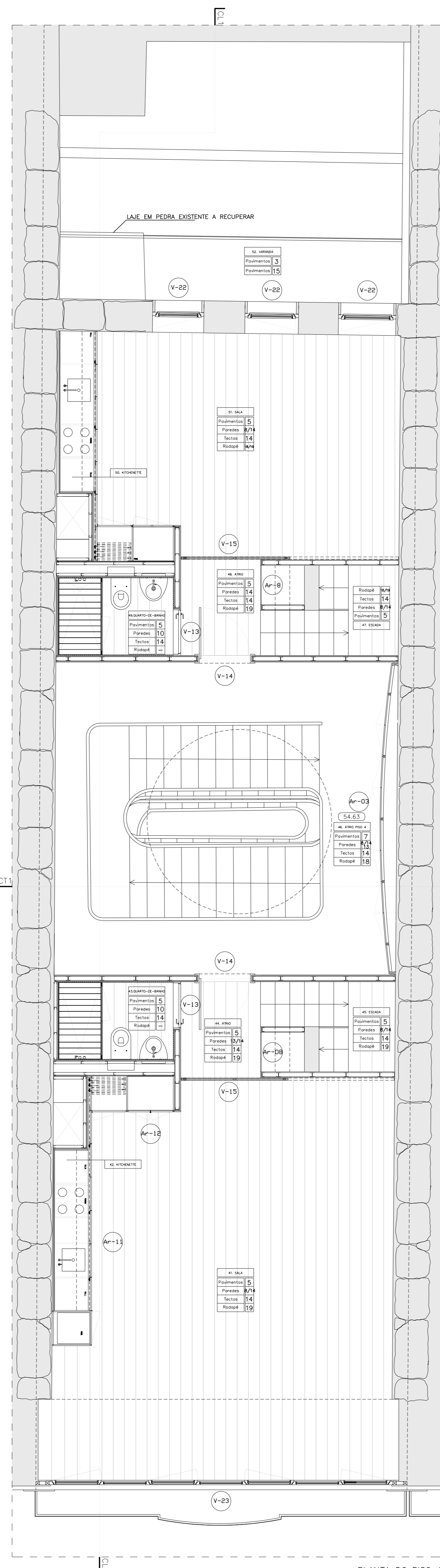
PLANTA DO PISO 4 À COTA 56.63
