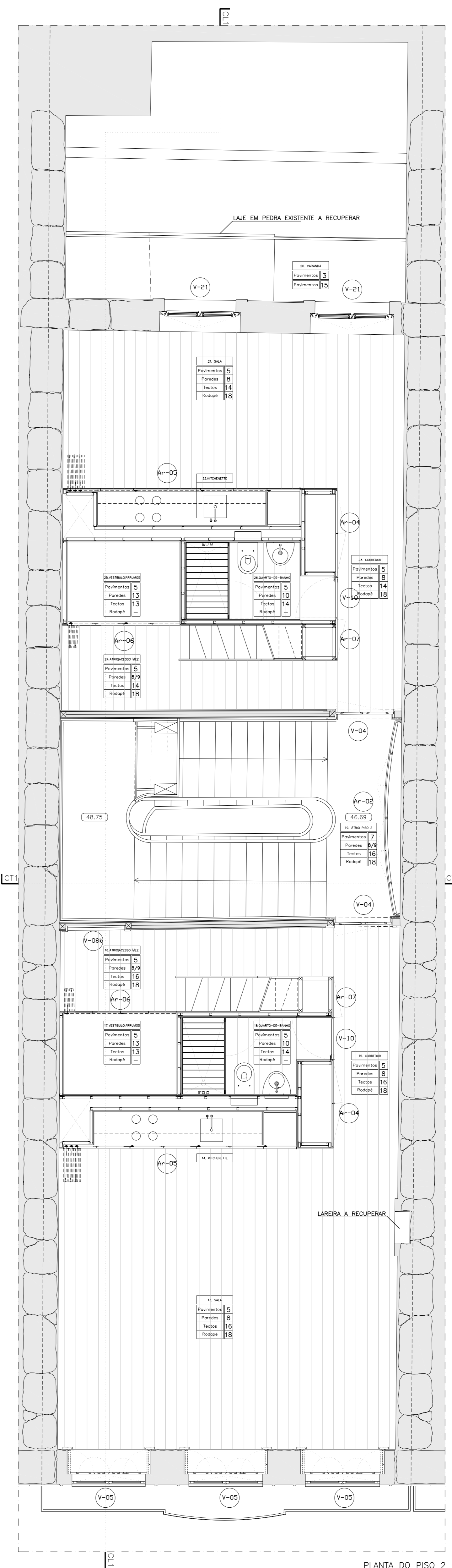
PLANTA DO PISO 2 A COTA 48.70
