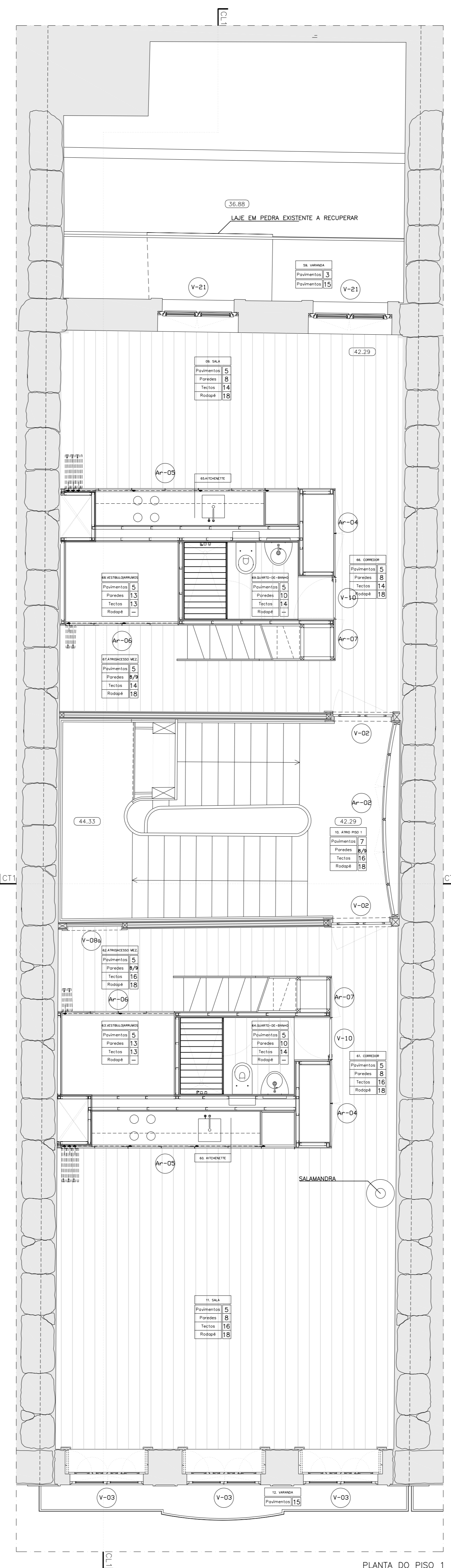
PLANTA DO PISO 1 A COTA 44.30
