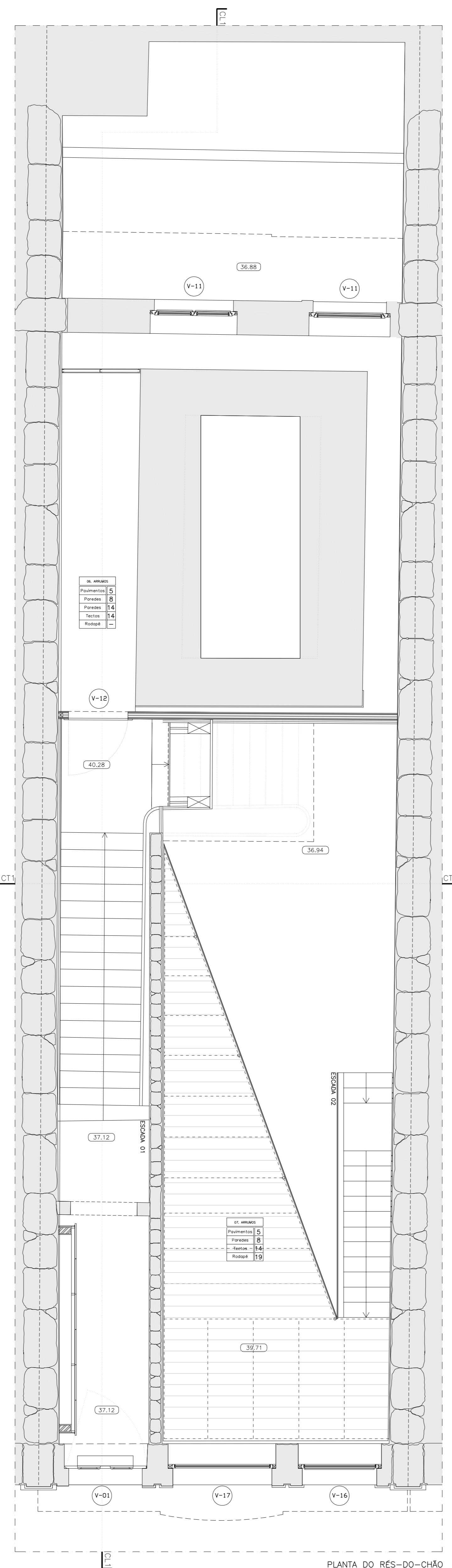
PLANTA DO RES-DO-CHÃO A COTA 40.60
