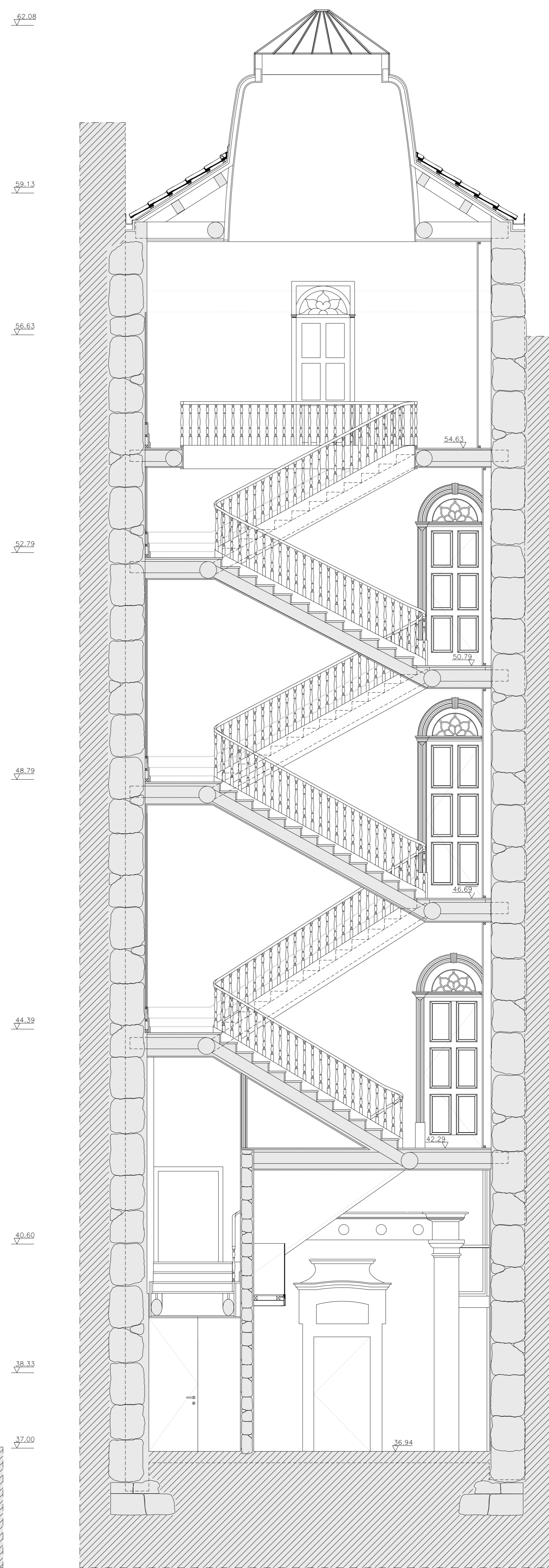
CORTE TRANSVERSAL CT1
