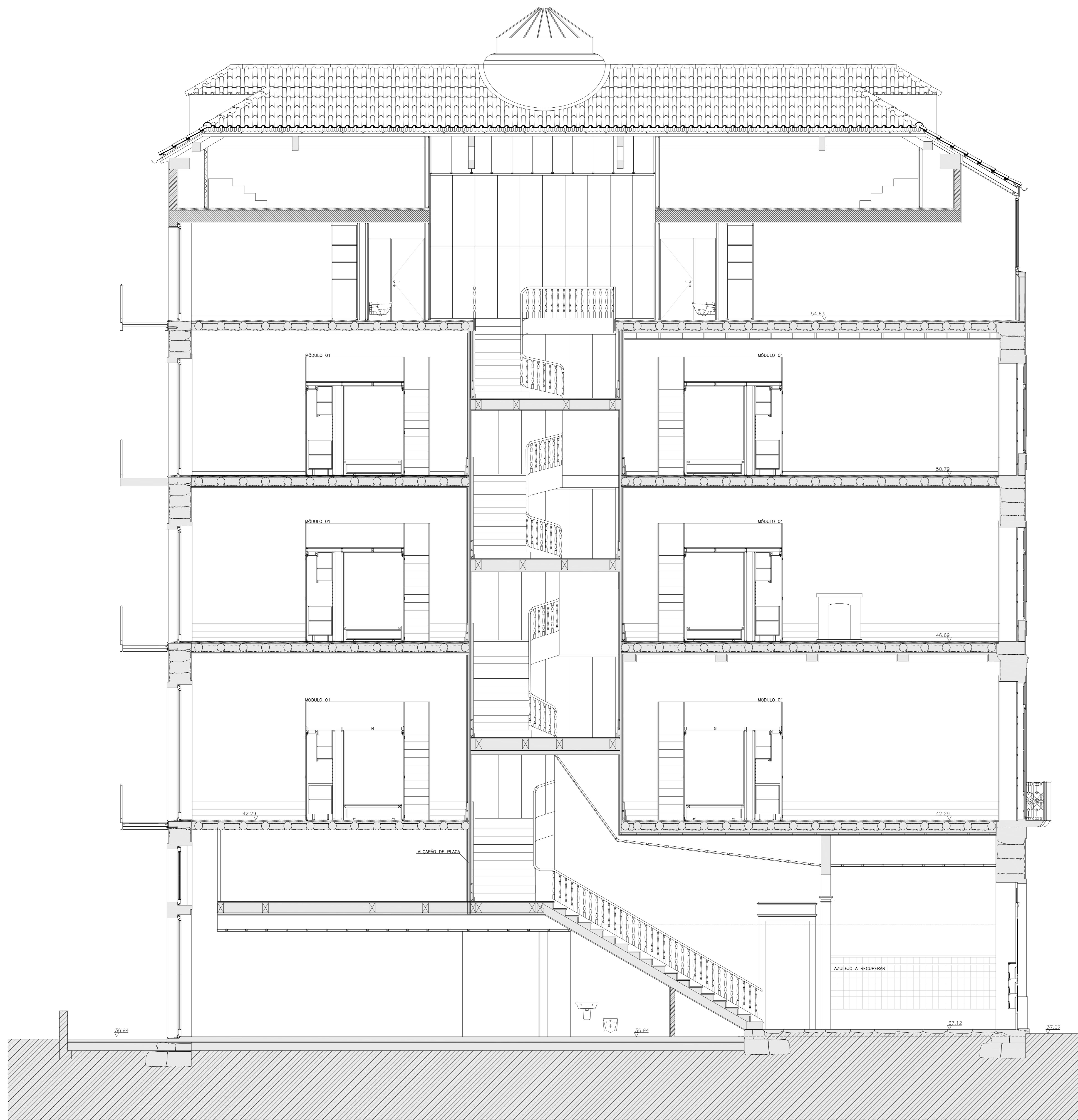
CORTE LONGITUDINAL CL 1
