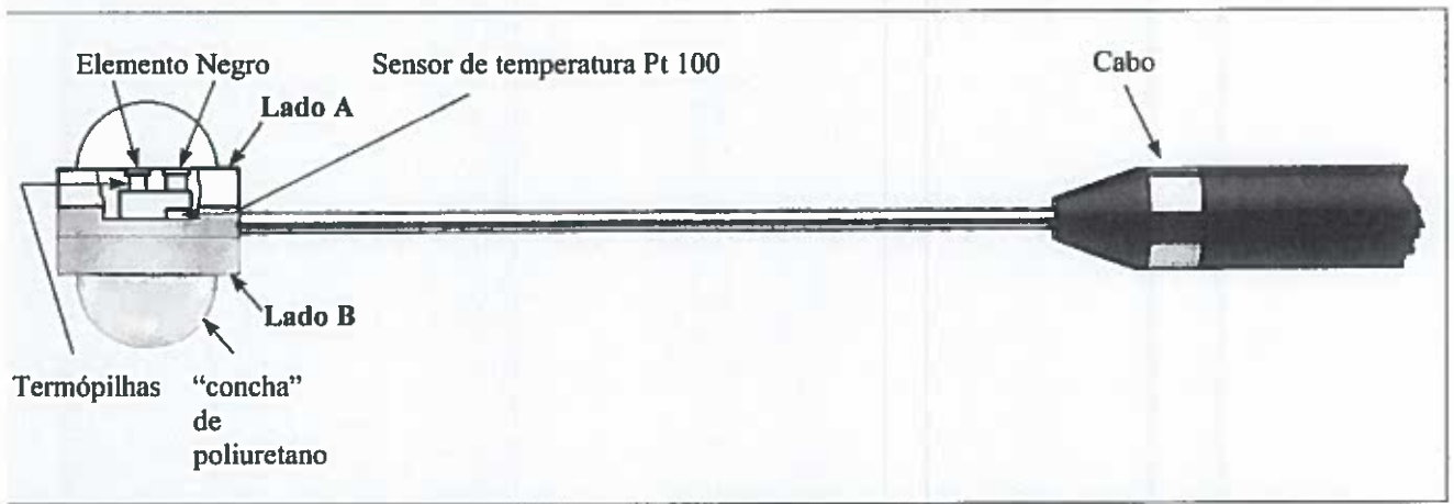
Figura J. 3. Sonda de Medição da Assimetria da Temperatura Radiante e da Temperatura Radiante Média. (Adaptado de: Bruel & Kjaer, 1990)
