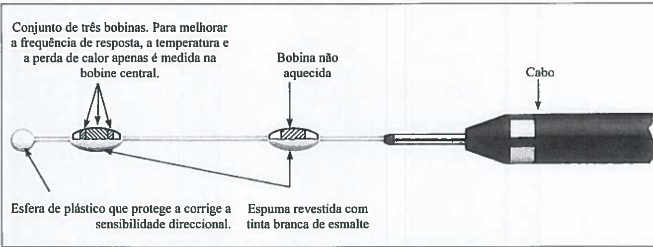
Figura J. 5. Transdutor de velocidade do ar. (Adaptado de: Bruel & Kjaer, 1990)
