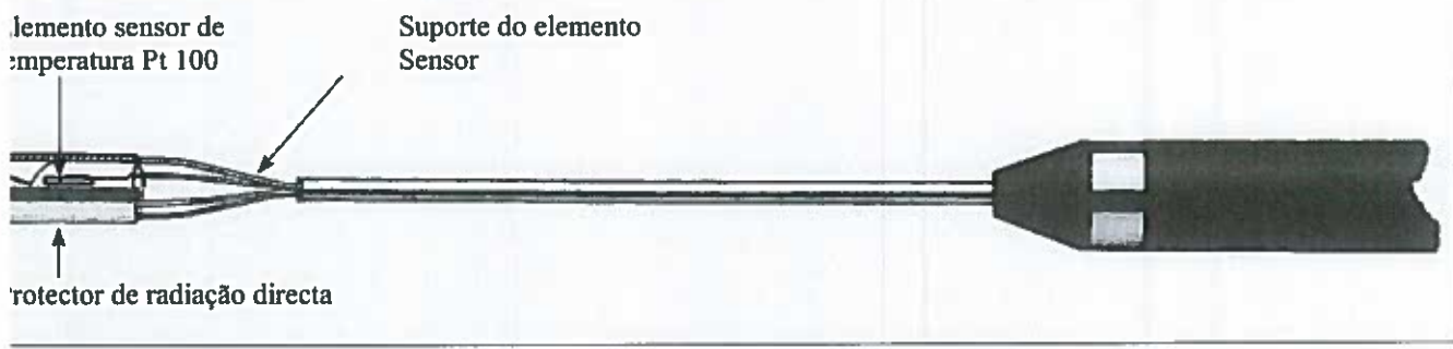
Figura J. 1. Sonda de medição da Temperatura do ar. (Adaptado de: Bruel & Kjaer, 1990)
