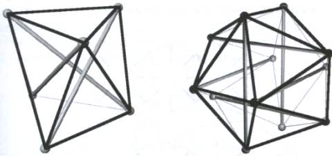
Figure 2.14. Enveloppes polyédriques des cellules à trois et six barres
