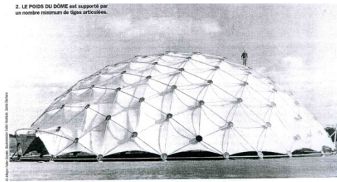
Figure 20 : Dôme géodésique. Le poids du dôme est supporté par un minimum de tiges articulées. Photos Allegra Fuller Snyder, Buckminster Fuller Institute, Santa Barbara, Inger scientific american, 1998b p.36
