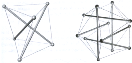
Figure 2.13. Cellules de tensegrité à trois et six barres
