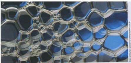
Figure 14 : La mousse de savon est une mousse topologiquement tridimensionnelle constituée de bulles. Les formes de la vie Pour la science. Juillet. Septembre. 2004 p.106
